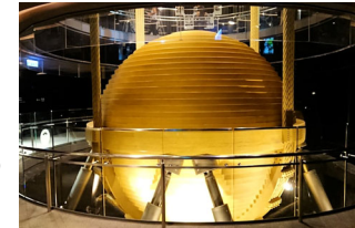
台北101制振装置のおもり(質量)
