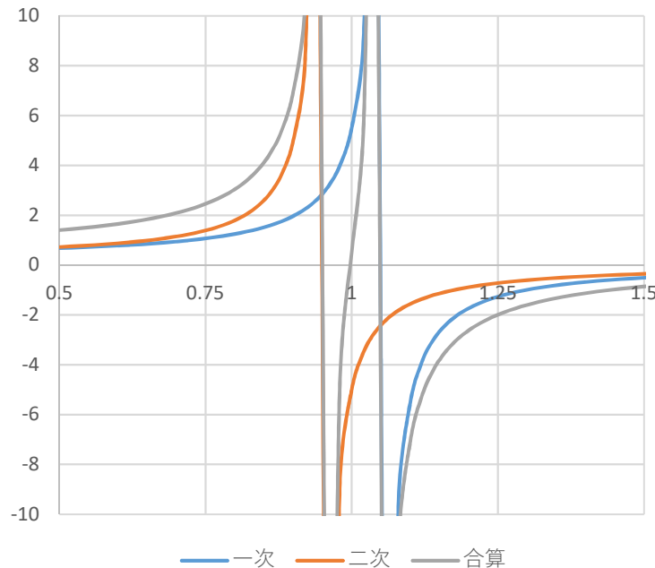
2自由度系の応答例
