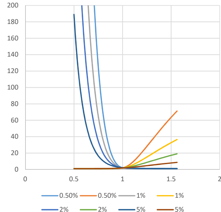
A=1の一般化質量
